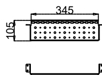
EM RF 05 20
