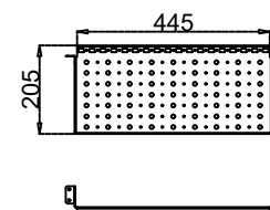
EM RF 06 30
