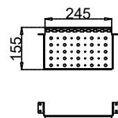
EM RF 04 25
