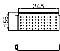
EM RF 05 25
