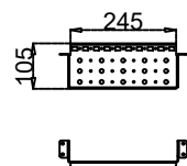
EM RF 04 20
