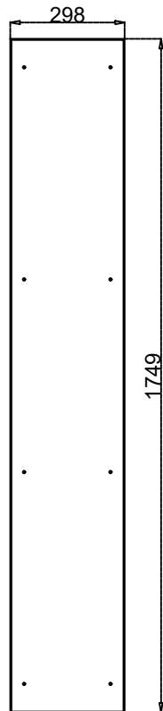
EFH SK 1803
